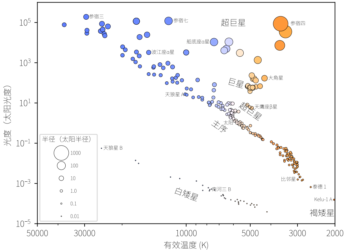
赫罗图
